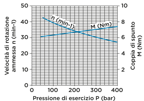
Velocità di rotazione n max. ammessa e relativa coppia di spunto M in funzione della pressione di esercizio P
